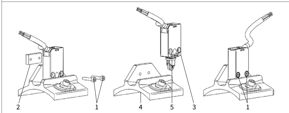
Rys. 13: Obracanie wyjścia kabla wyłącznika krańcowego
