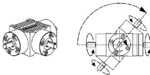
Abb. 8: T-Ausführung (Kegelradgetriebe)
