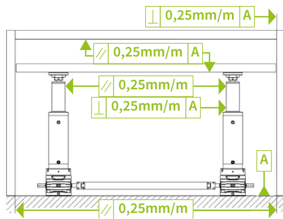
Abb. 6: Einbaugenauigkeit: Parallelität und Rechtwinkligkeit
